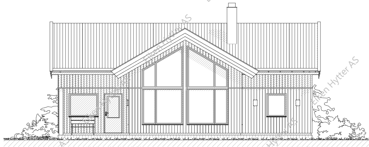
Fasade 1
