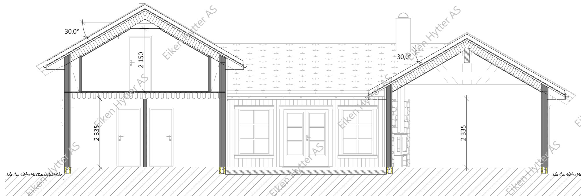
Snitt - A
