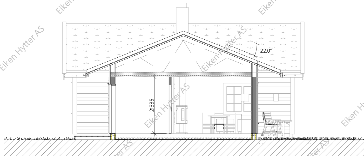
Snitt - B
