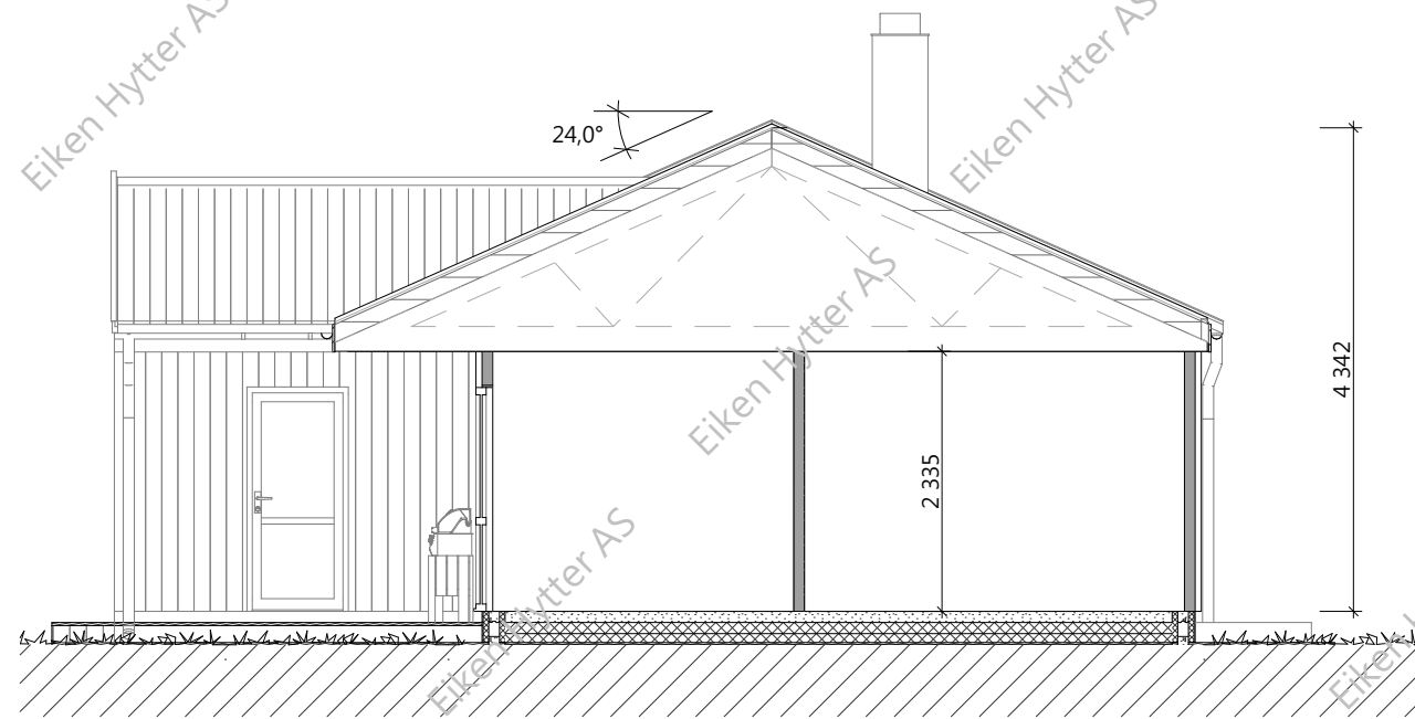
Snitt BB
