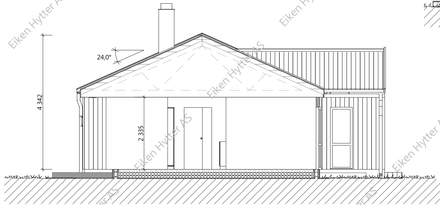
Snitt AA
