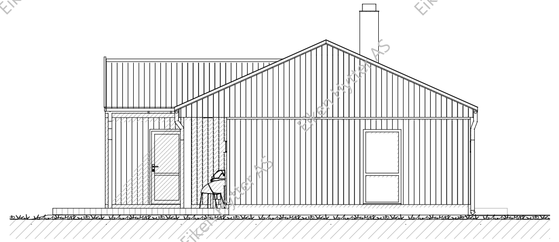
Fasade 4
