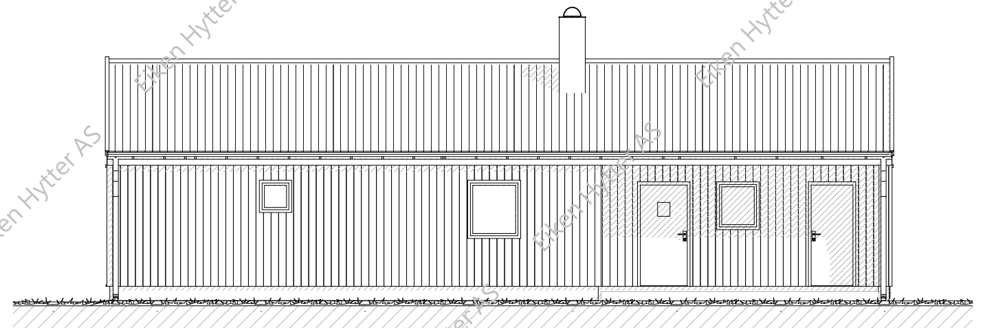
Fasade 2
